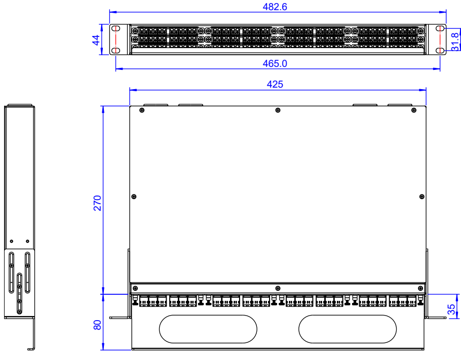
图 2.5 1U 机箱 144 芯
