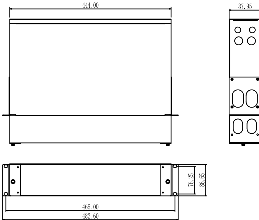
图 2.2 2U 机箱
