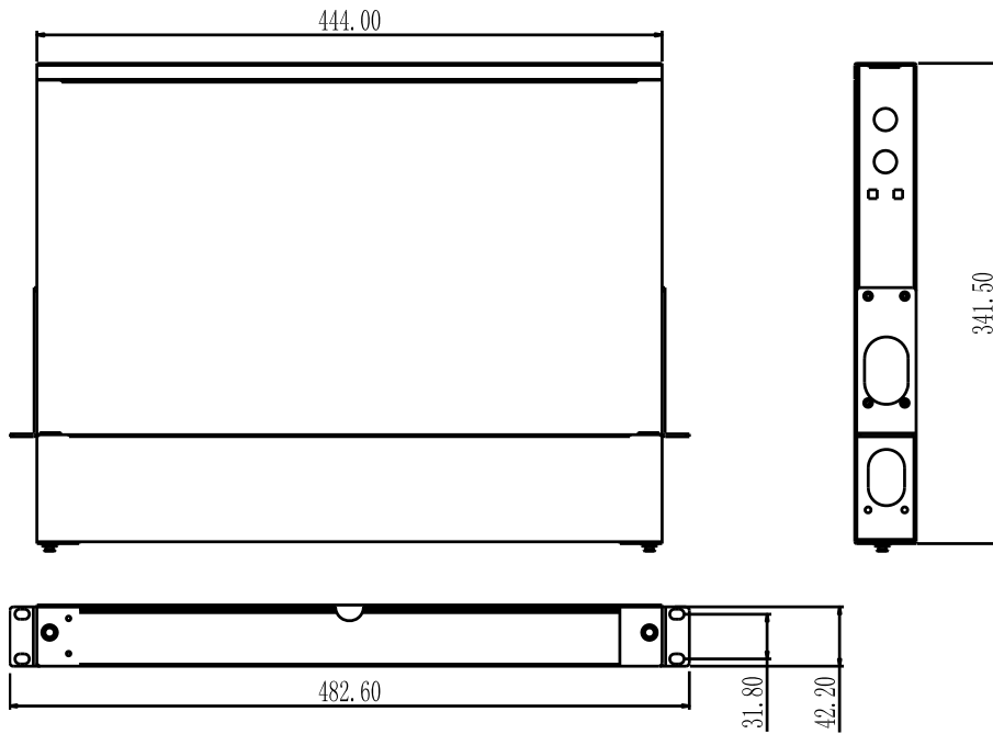
图 2.1 1U 机箱
