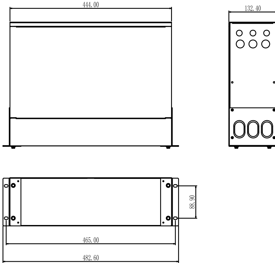
图 2.3 3U 机箱
