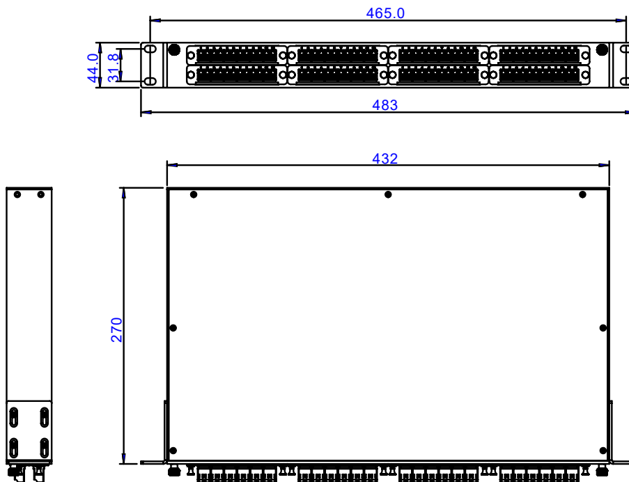
图 2.4 1U 机箱带导轨
